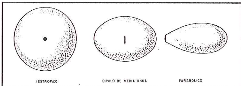
Figura 1. Representación teórica del diagrama de radiación de las siguientes antenas: isotrópica, dipolo de media onda y reflector parabólico.
